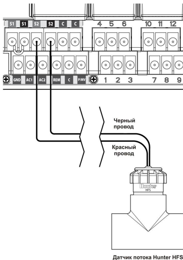
Датчик потока Hunter HFS
