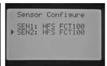
SEN 1 и 2 датчик потока (HFS FCT100)
